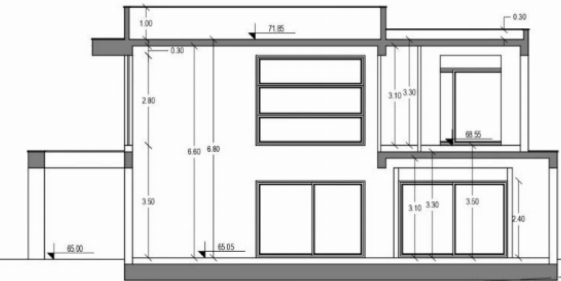
TOMH A-A' ΚΛΙΜΑΚΑ 1:100
