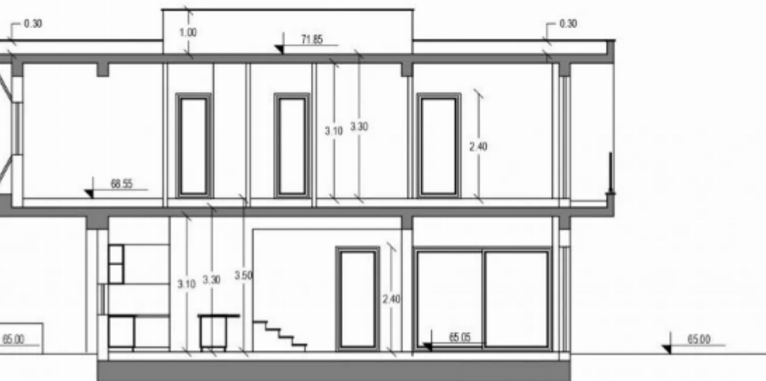
TOMH B-B' ΚΛΙΜΑΚΑ 1:100
