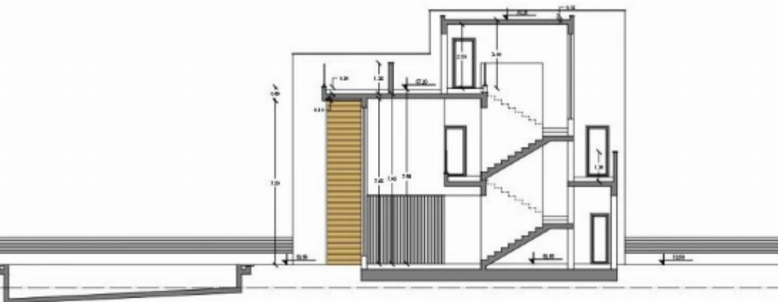
TOMH A-A K/M/MAKA 1.200
